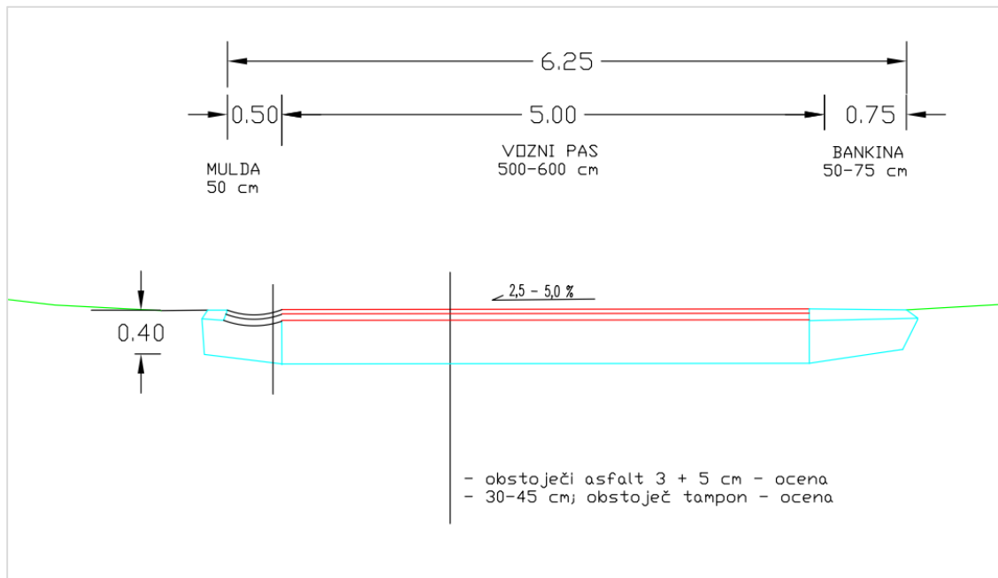
Slika 8: Karakteristični prerez – obstoječe stanje
