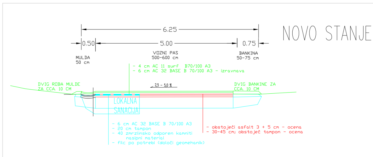
Slika 10: Karakteristični prerez – novo stanje
