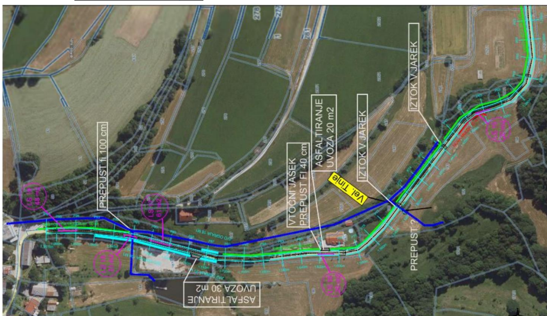
Slika 13: Gradbeni situacija 3
