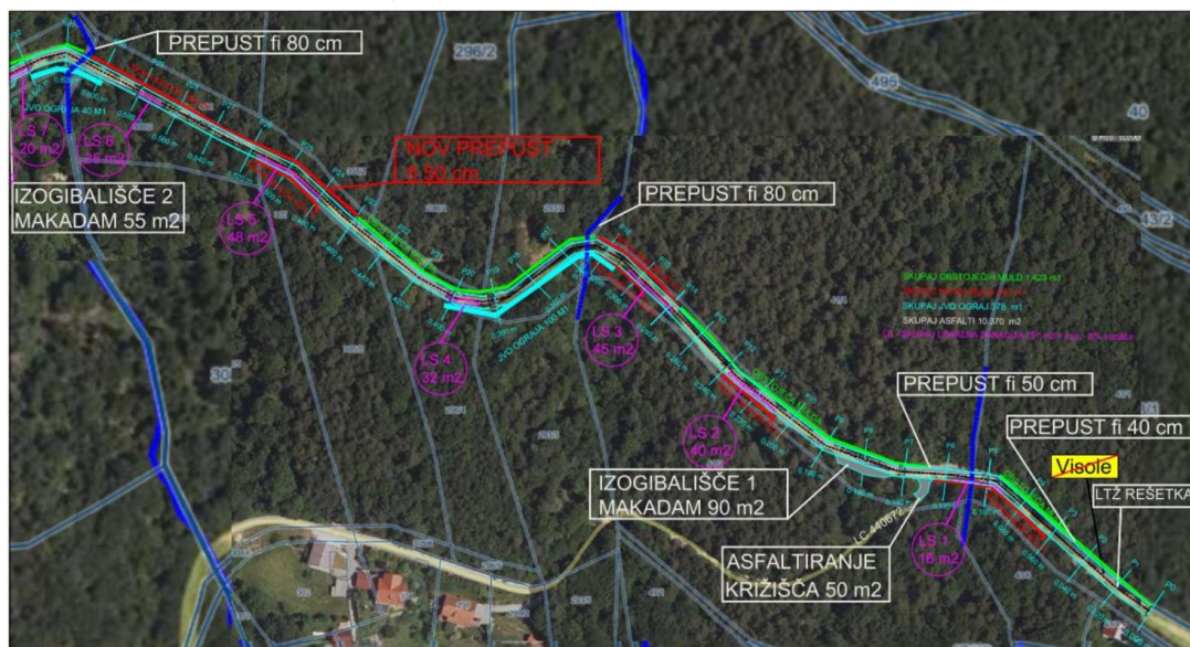
Slika 11: Gradben situacija 1
